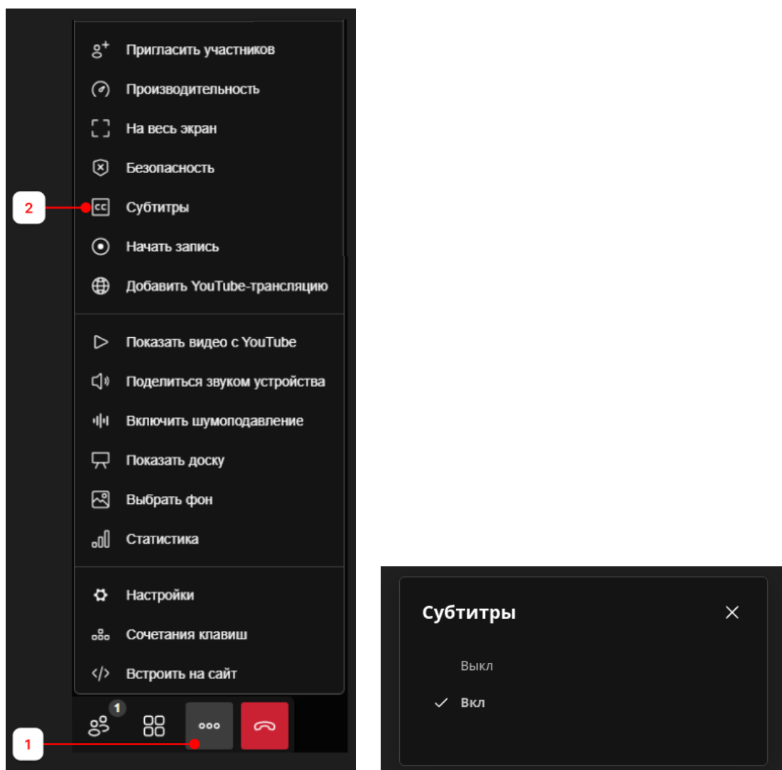
Рисунок 12 — Включение транскрипции
