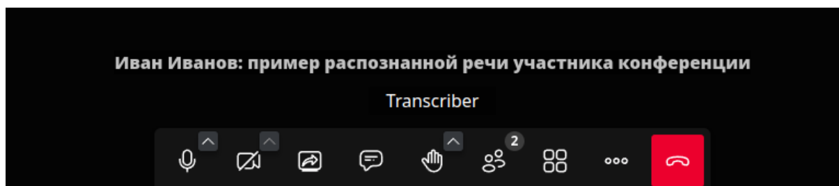
Рисунок 11 — Функция транскрипции
